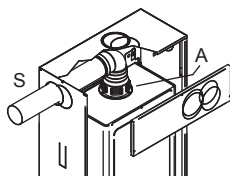
Esempi di sistemi con aspirazione diretta B_{22}
