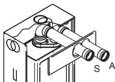
Esempi di sistemi con aspirazione diretta B_{22}
