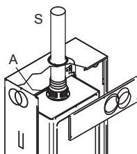
Esempi di sistemi con aspirazione diretta B_{22}
