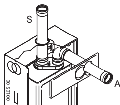
Esempi di sistemi separati C_{42} , C_{52} , C_{82} , C_{92}
